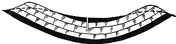
चित्र १४८—आर्टीजियन कुएँ।
